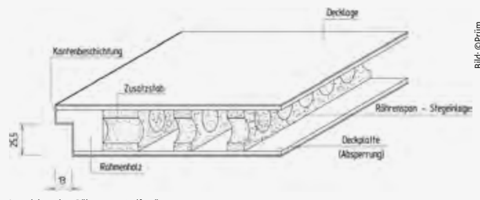
Innenleben einer Röhrenspanstreifentür
