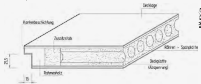
Innenleben einer Röhrenspanplattentür
